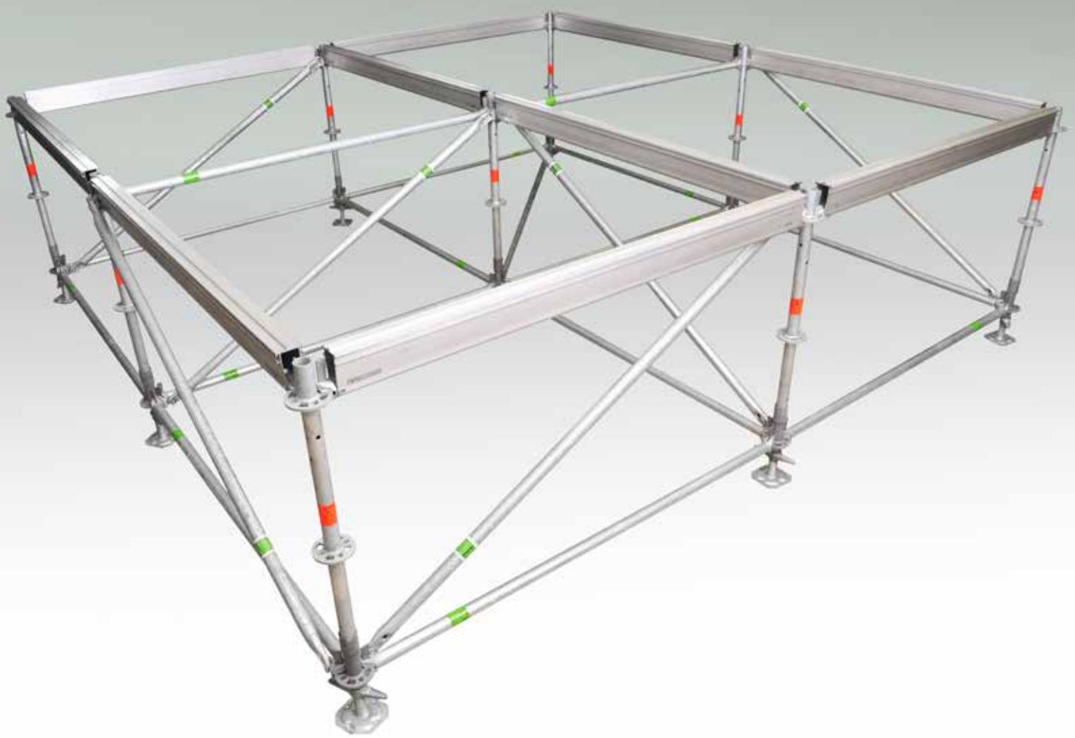
Lastenträgerbühnen bis 300 cm in Verbindung mit Layher-Allround-Metric-Gerüstsystem in Stahl im Raster 200 x 200
